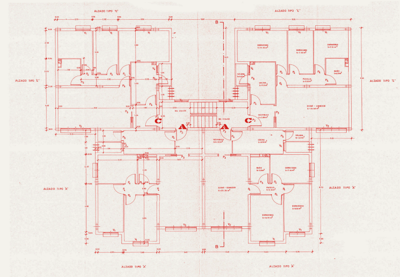
Bloque A: planta tipo
